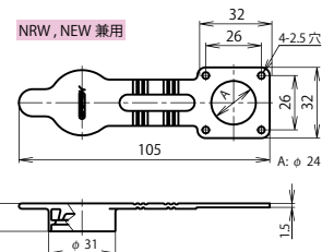
レセプタクルゴムキャップ: NRW-24-RCa・2
