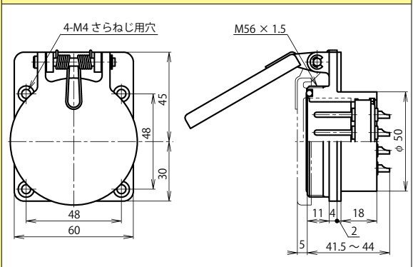
キャップ付きレセプタクル: NT-50 ■ -CRM
