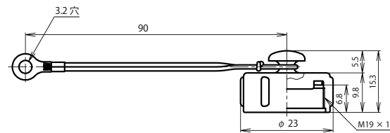
レセプタクルキャップ: PLW-14-RCa
