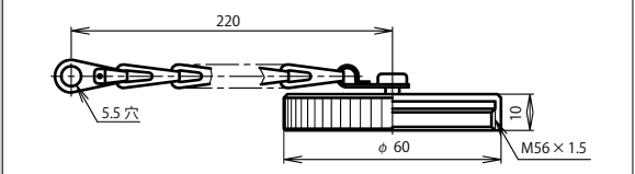
レセプタクルキャップ: NT-50-RCa
