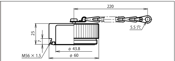
プラグキャップ: NT-50-PCa
