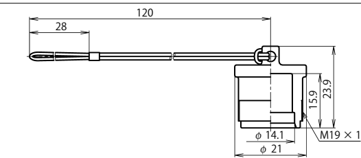
プラグキャップ: PLW-14-PCa
