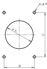
角フランジレセプタクル（縦長4点穴）
