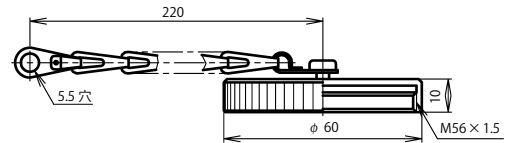
レセプタクルキャップ: NT-50-RCa
