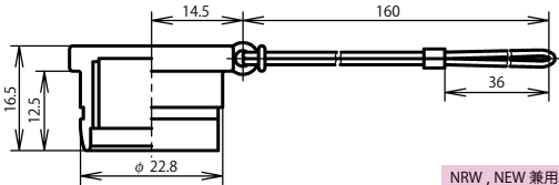
プラグ防水キャップ: NRW-20-PCa・1
