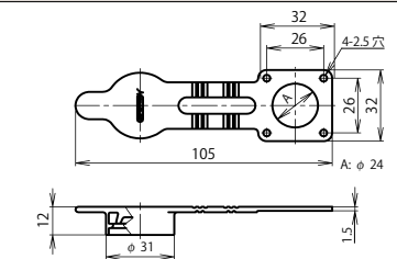
レセプタクルゴムキャップ: NRW-24-RCa・2
