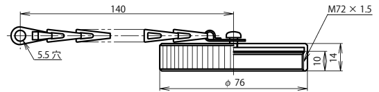
レセプタクルキャップ：64EUMW-RCa
