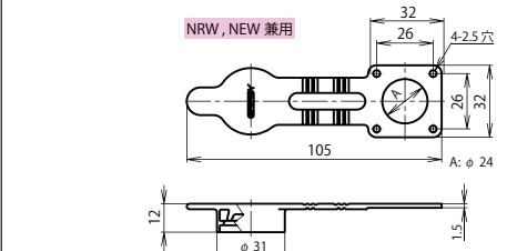
レセプタクルゴムキャップ: NRW-24-RCa・2
