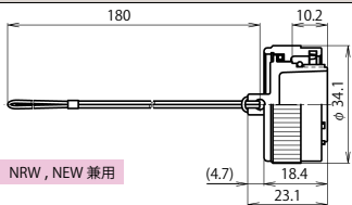
アダプタ防水キャップ: NRW-24-AdCa・1
